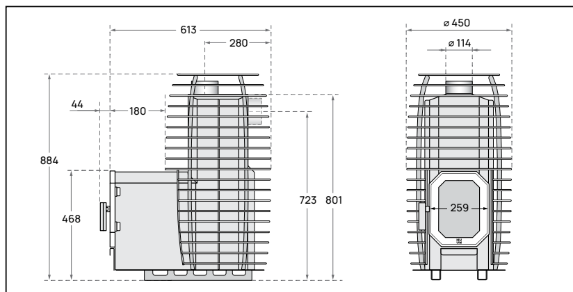
Slika 4. Dimenzije peći za saunu HIVE Flow Mini LS.
