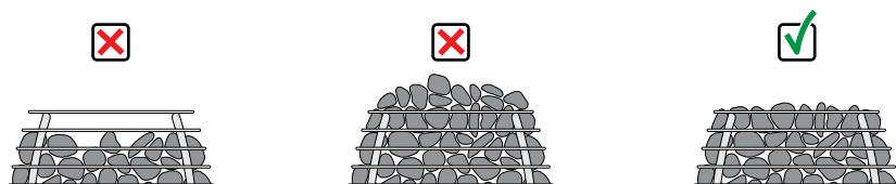
Figura 14. Colocación de las piedras de HIVE Flow.
