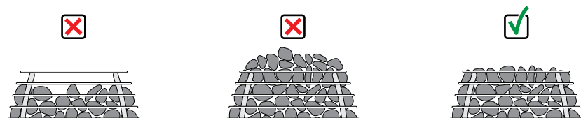
14. ábra. A HIVE Flow kövek lerakása.
