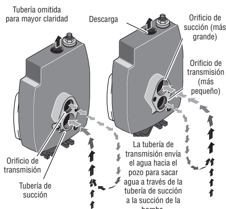
Figura 2 - Funciones de Succión y Transmisión
