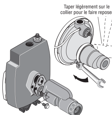
Figure 4 - Montage de l'éjecteur - puits peu profonds
