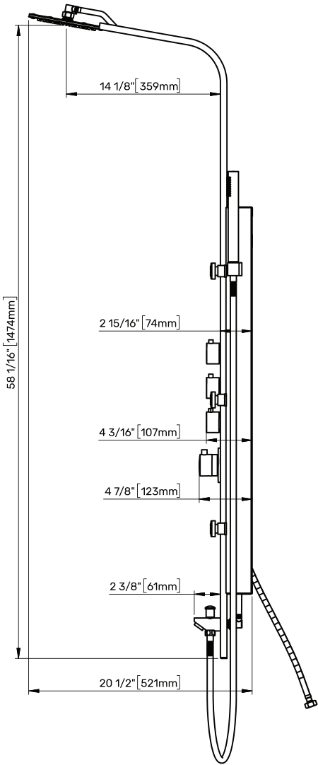
SIDE VIEW / VISTA LATERAL / VUE DE CÔTÉ
