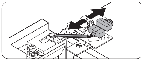
Platte schroevendraaier
