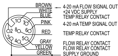
CT wiring
