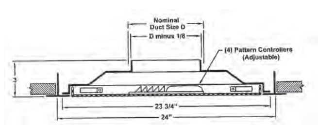
PAS3F (Standard Lay-In)
