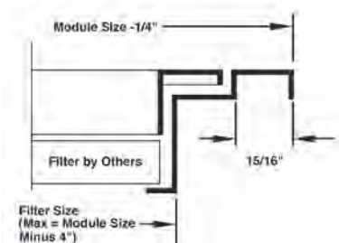
50FF1 T-Bar (Lay-In)
