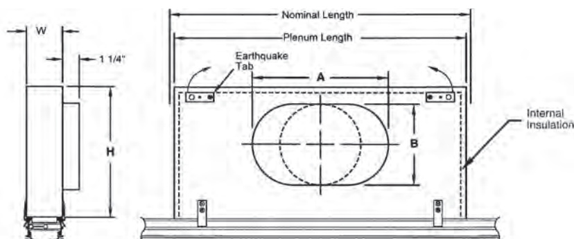
FBPI Plenums
