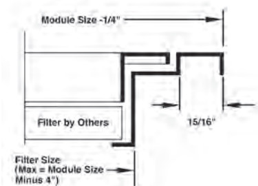
350RLF1 T-Bar (Lay-In)
