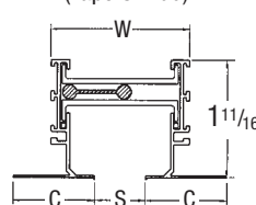
Border Type 22 (Tape & Mud)
