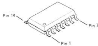
μPD4066BG (Q1077)
