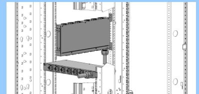
bPDU G2 の 1U および 0U での取り付け
