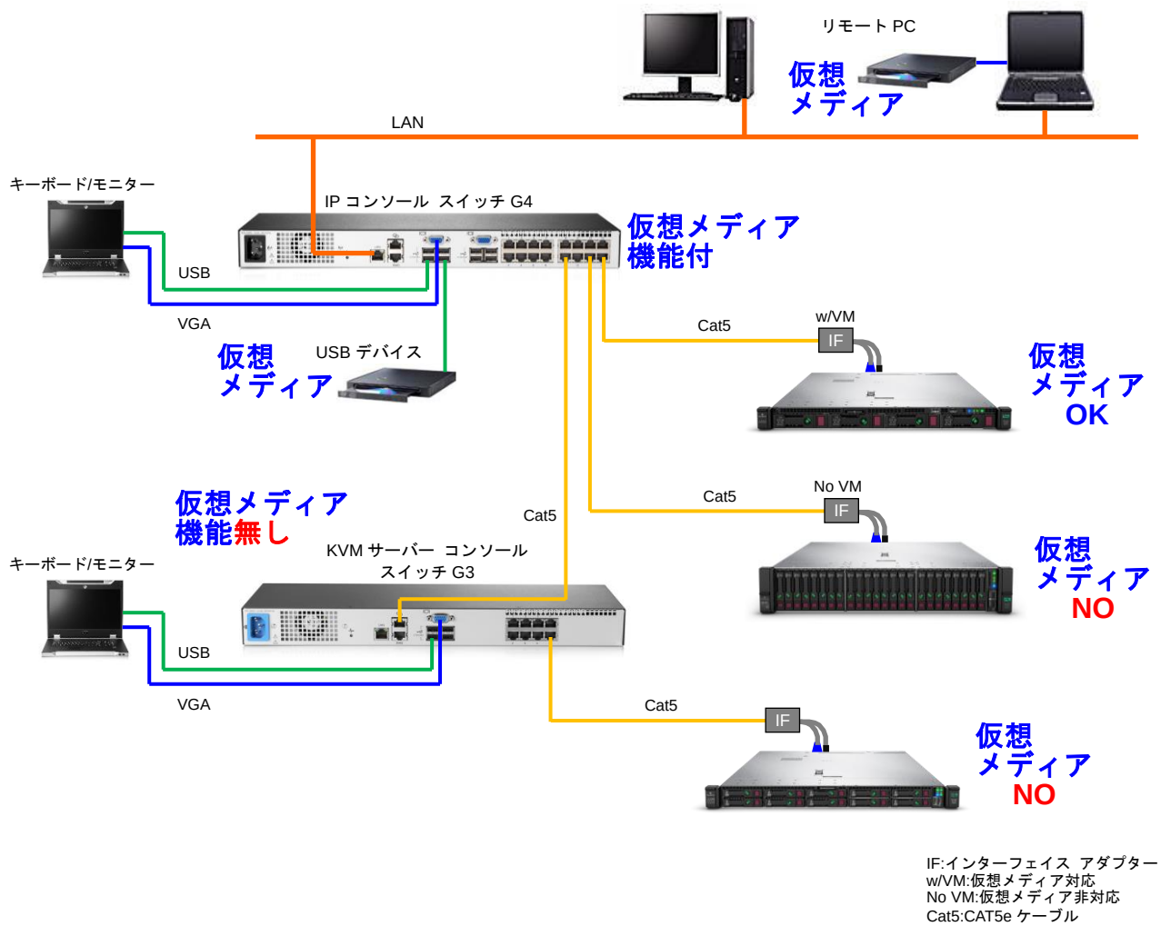
IP コンソール スイッチ G4 仮想メディア機能付の各サーバー、スイッチのカスケード接続、仮想メディア機能の論理的接続イメージ
