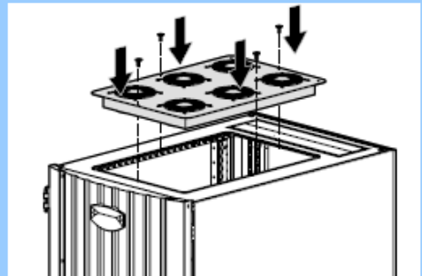
ラックファン キット
