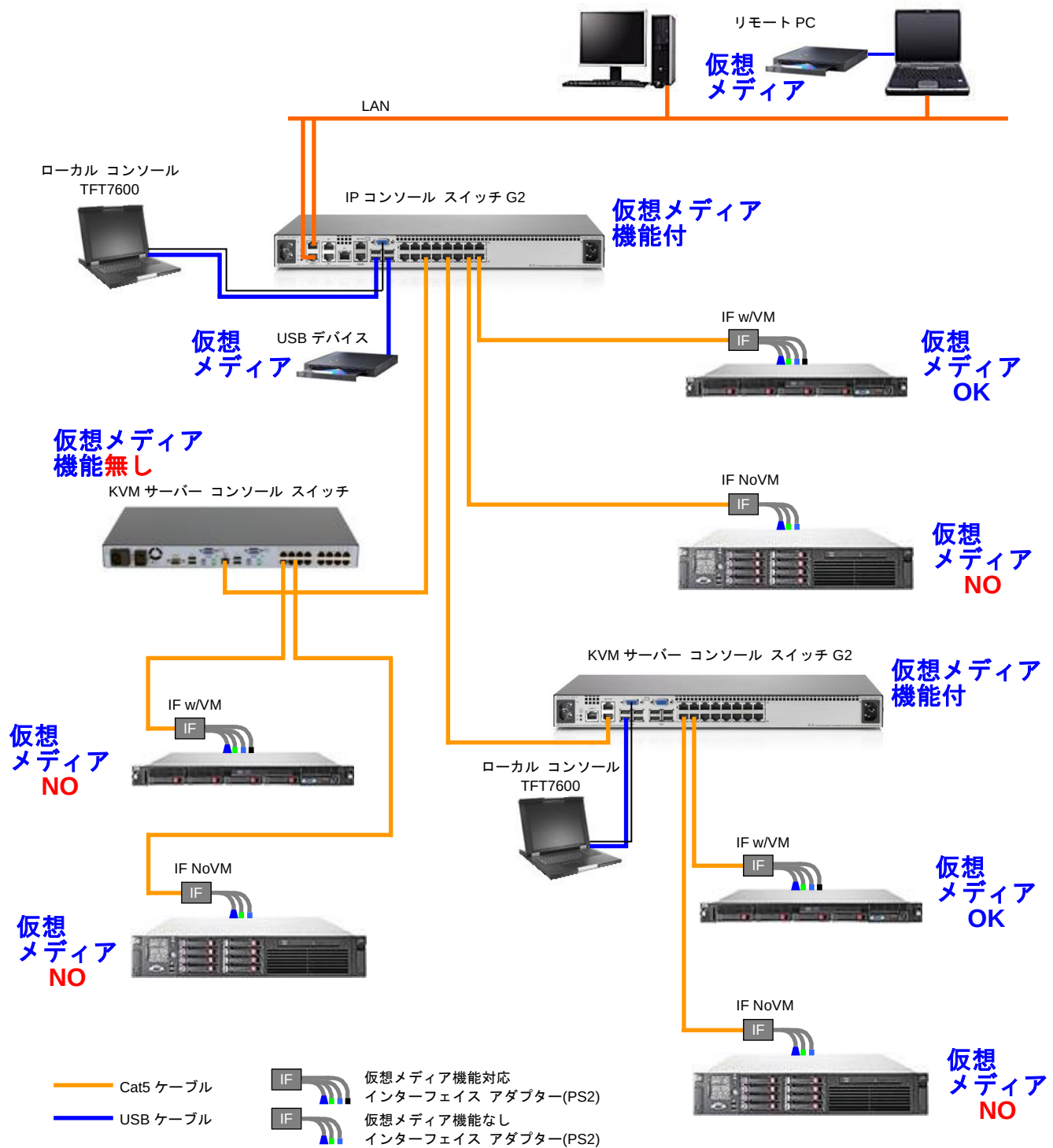
IP コンソール スイッチ G2 仮想メディア機能付の各サーバー、スイッチのカスケード接続、仮想メディア機能の論理的接続イメージ
