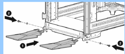
ラック固定脚セット(600W 高重量用 ver.2)の取付け
