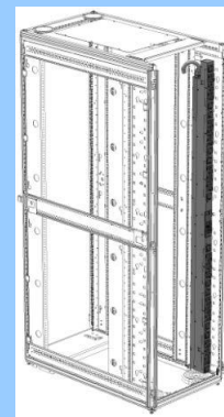
ボタンを利用した垂直マウント型フルハイト 高密度 PDU の取り付け(図は 42U ラック)
