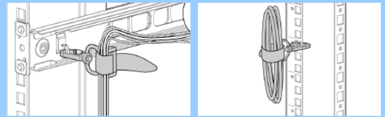
ケーブル マネジメント(クリップ付ストラップ)キットの利用例
