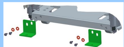
ラック固定キットの取付け(ラック前面)
