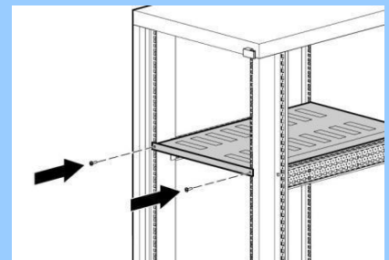
モニタ シェルフ キット
