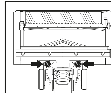
RIMOZIONE DEL TERGIPAVIMENTO
