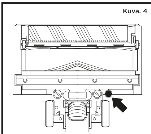
FLOORDETECT- LATTIANTUNNISTUSANTURI
