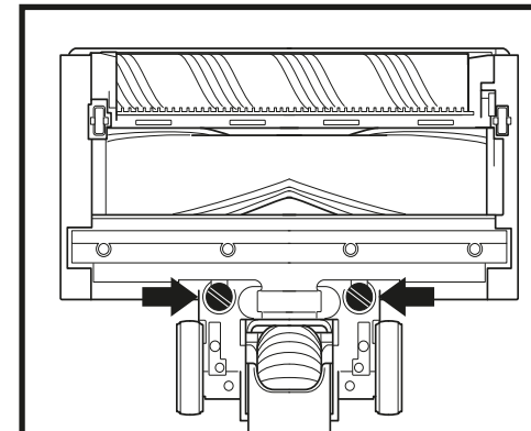
VEDENPURISTUSTELAN IRROTTAMINEN
