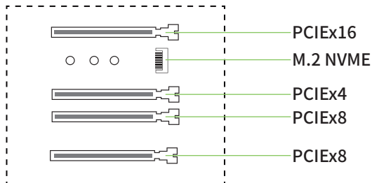
图2-4 PCI扩展插槽
