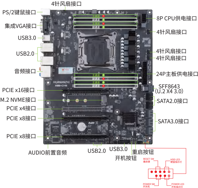
图1-1 X99-CH8主板图解
