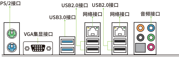
图1-2 整体后置I/O面板展示
