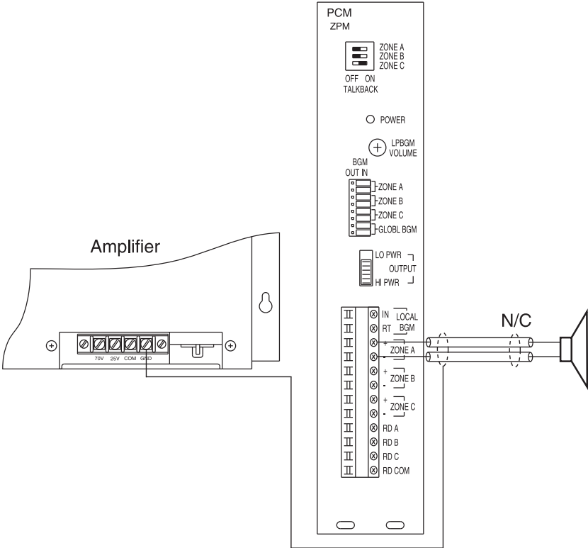
Zone Wiring
