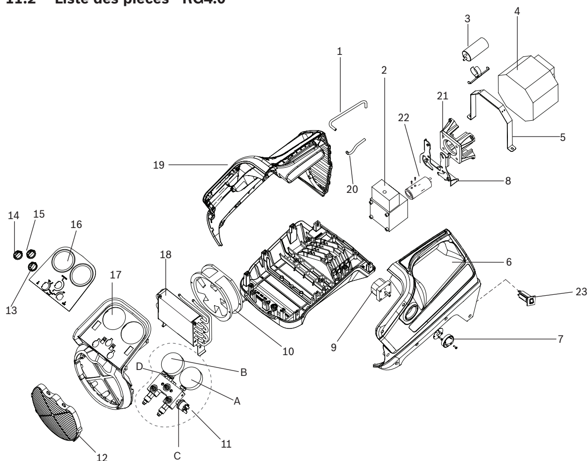
Fig. 6: Éclaté de l'unité RG4.0
