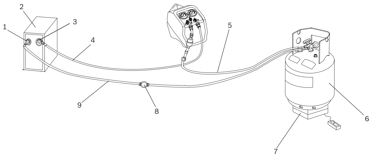
Fig. 2: Recupero push/pull
