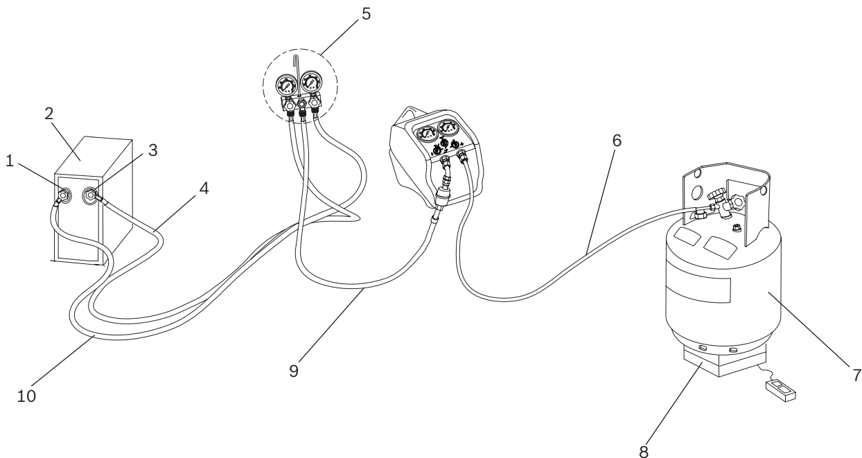
Fig. 3: Recuperación normal
