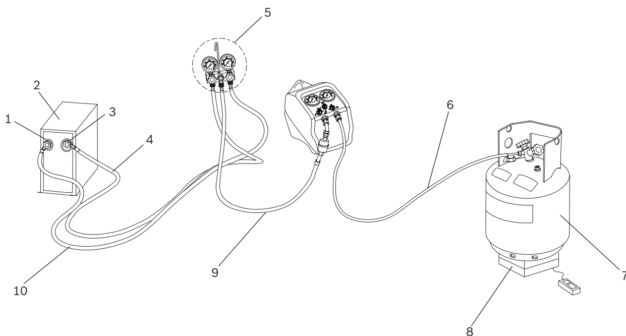
Fig. 5: Recupero normale
