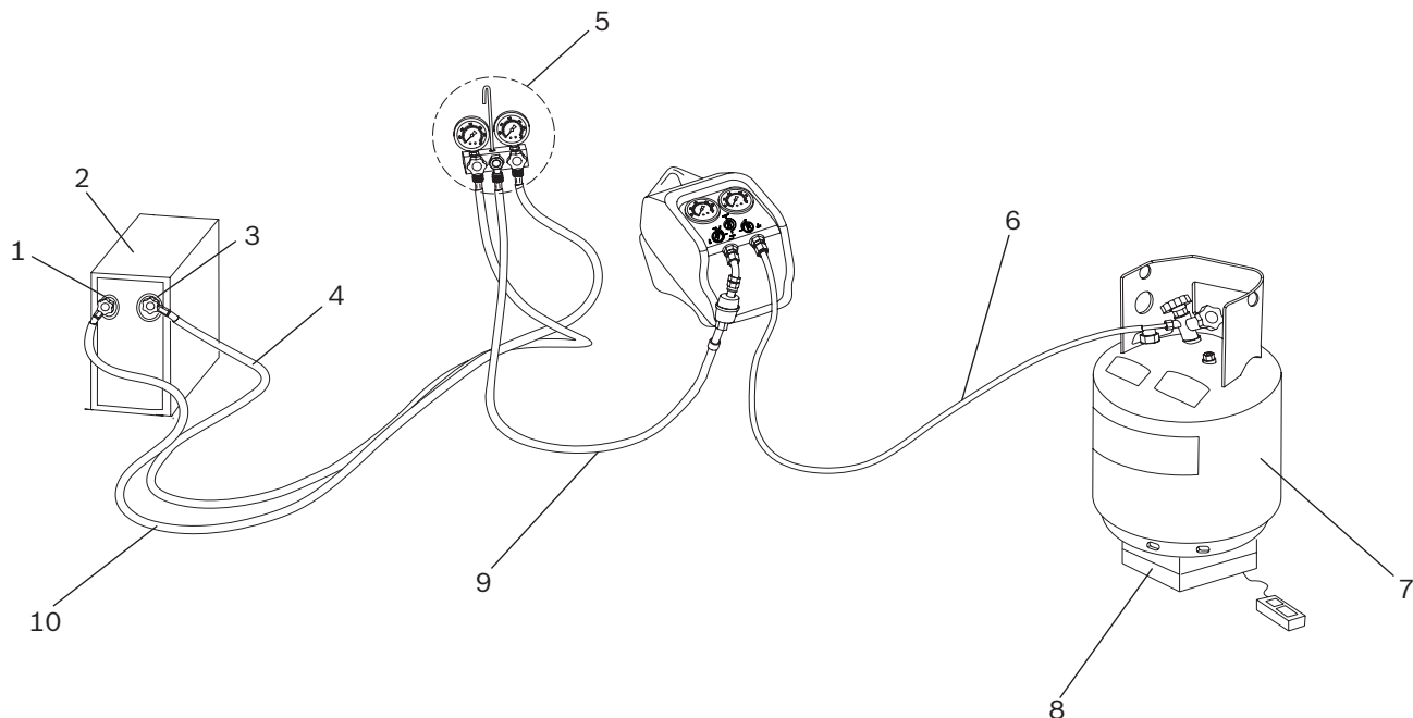
Bild 3: Normal återvinning
