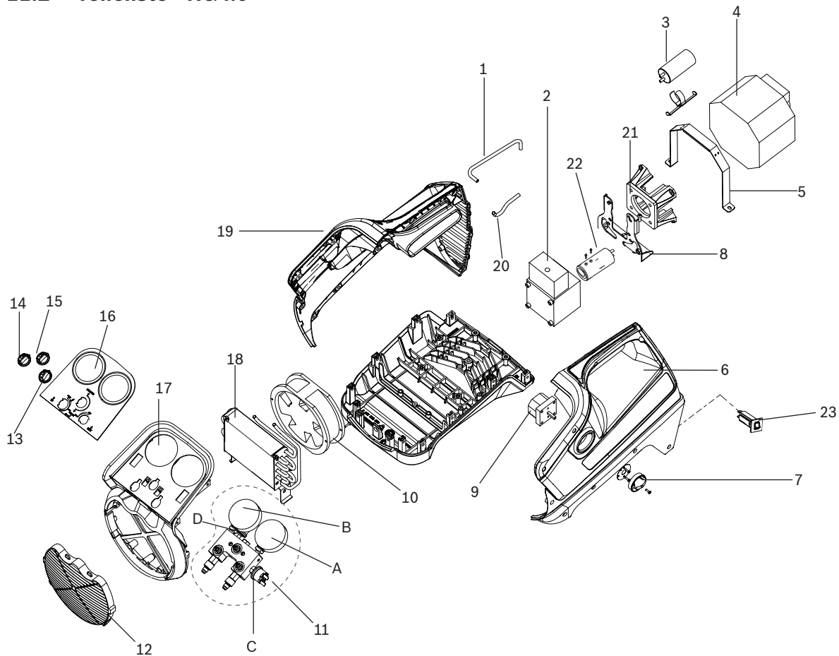
Abb. 7: Explosionsdarstellung - RG4.0
