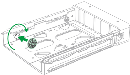
从尾端内侧装入，按顺时针方向旋转使其卡紧
