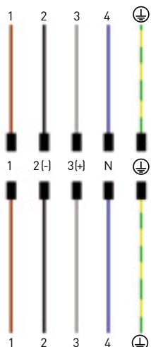
RETTBOX® 20 A/400V
