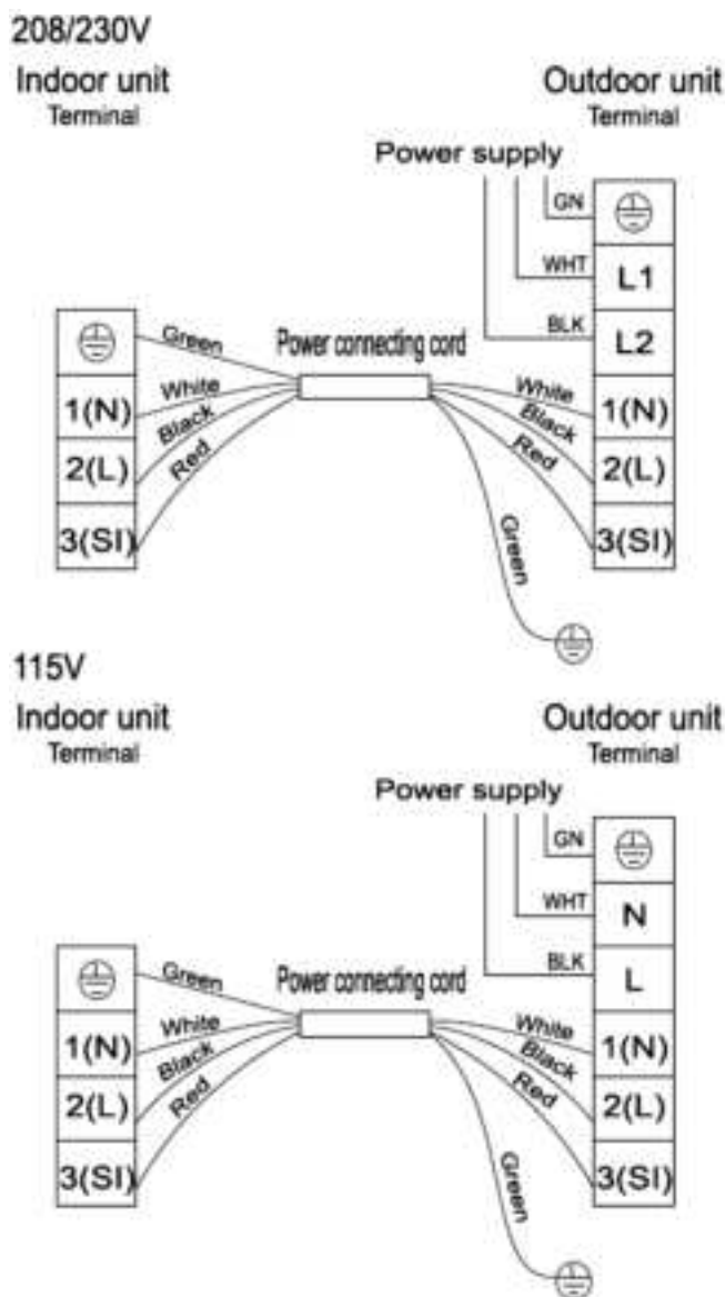
Fig. 4.4b: Diagrama de cableado
