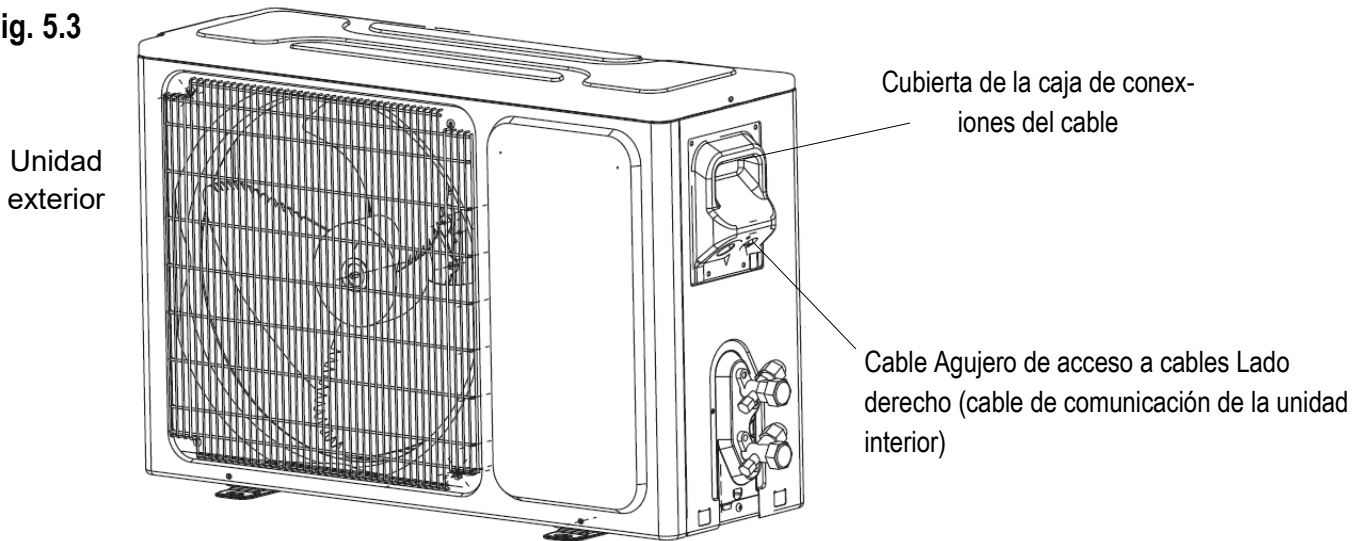
Fig. 5.3b: Conexiones del cable de comunicación
