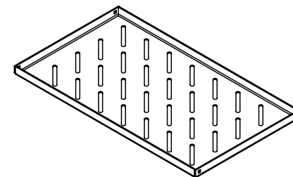
BOTTOM PAN
