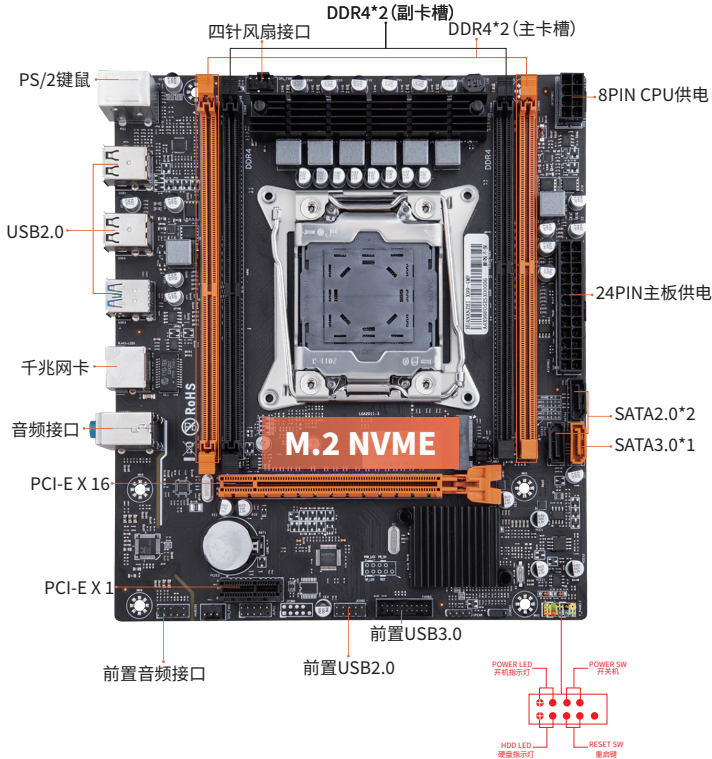
图1-1 X99-4MF主板图解
