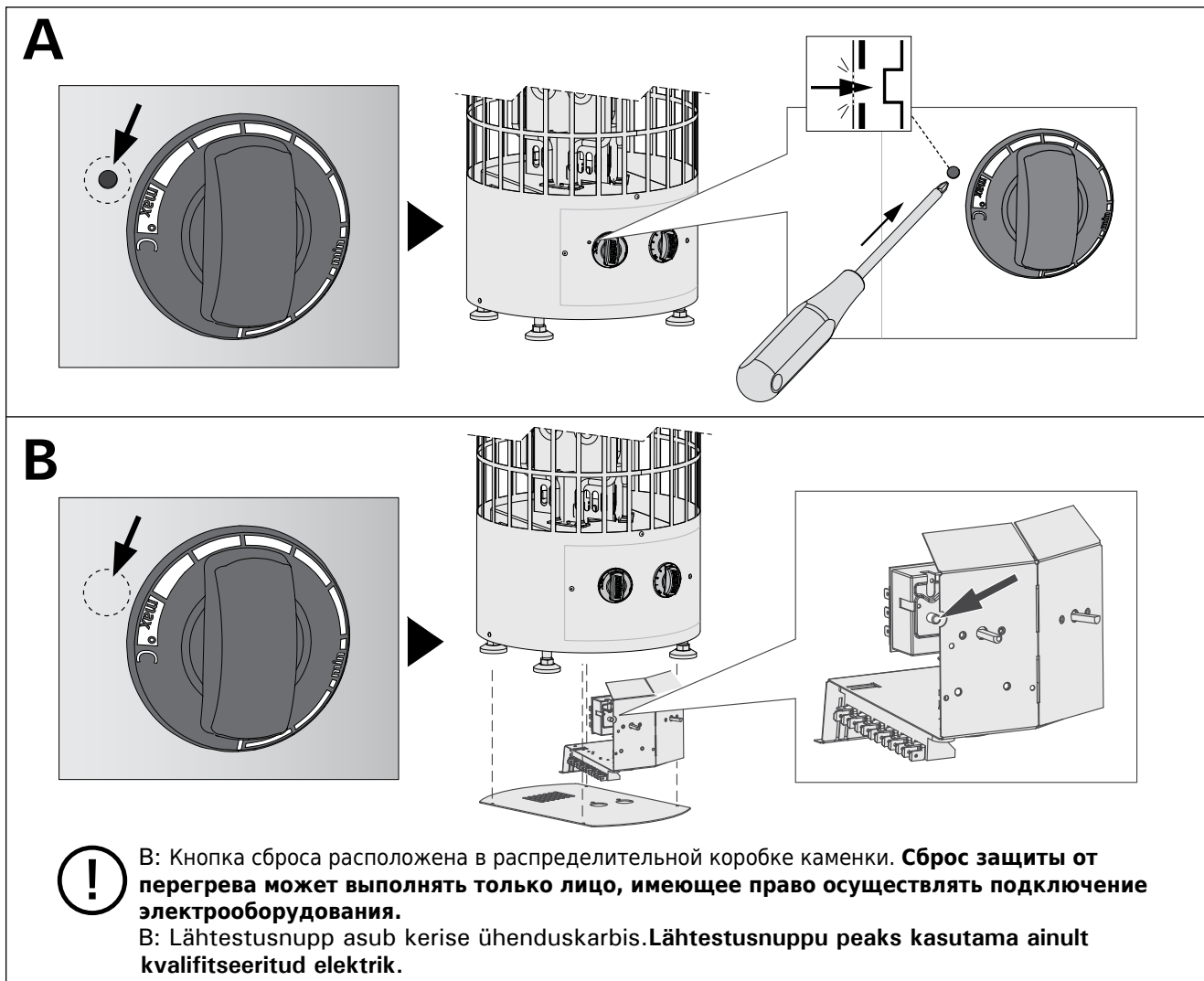
Рисунок 10. Кнопка сброса защиты от перегрева
