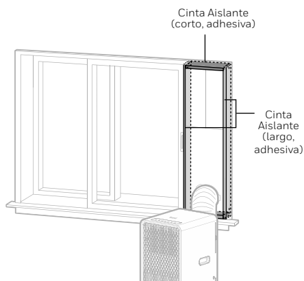
Ventana corrediza horizontal
