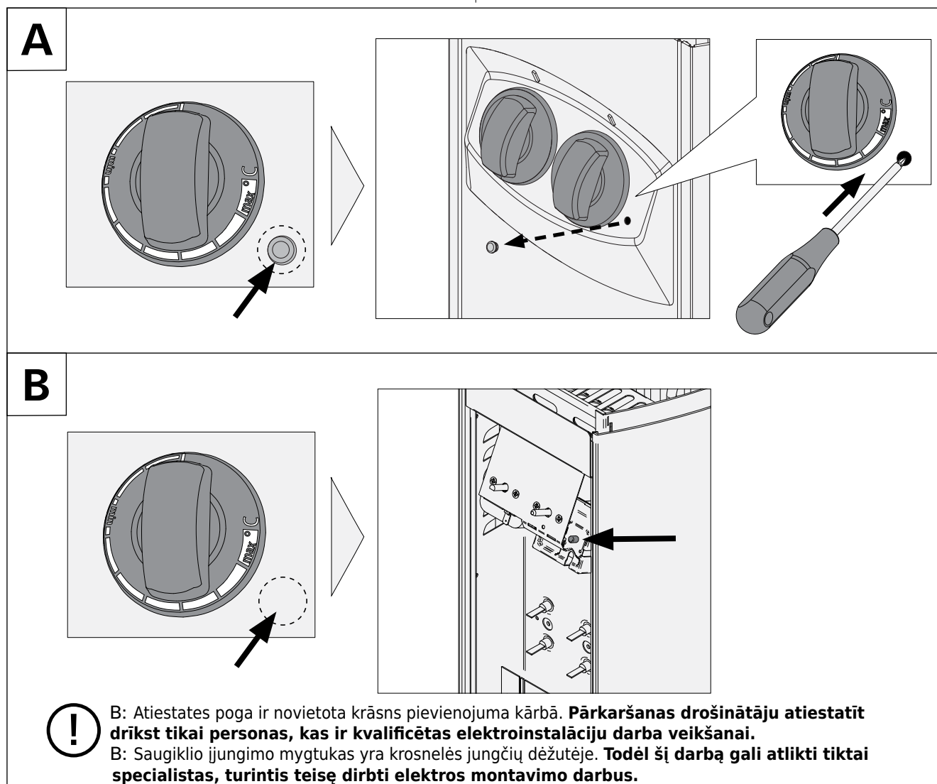
9. zīm. Pārkaršanas drošinātāja ieslēgšanas poga 9 pav. Perkaitimo saugiklio įjungimo mygtukas
