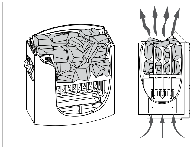
Rys. 1. Układanie kamieni w piecu Obrázek 1. Skládání kamenů
