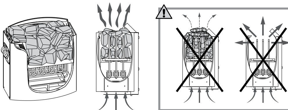
Figure 1. Mise en place des pierres du poêle Figuur 1. Saunastenen opstapelen
