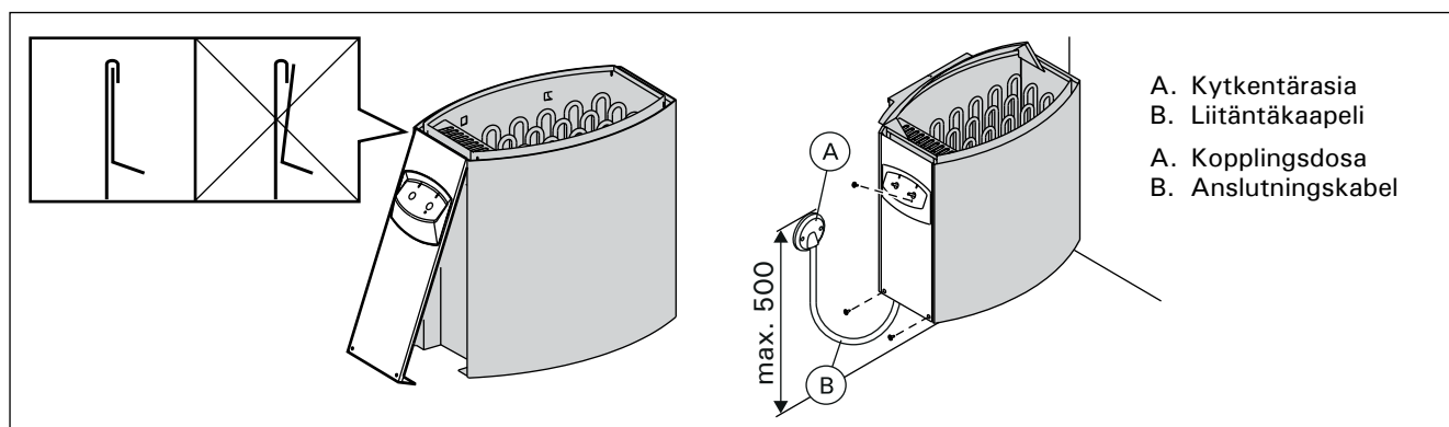
Kuva 8. Kytkentäkotelon kannen sulkeminen (mitat millimetreinä) Bild 8. Stänga anslutningshusets front (mått i millimeter)
