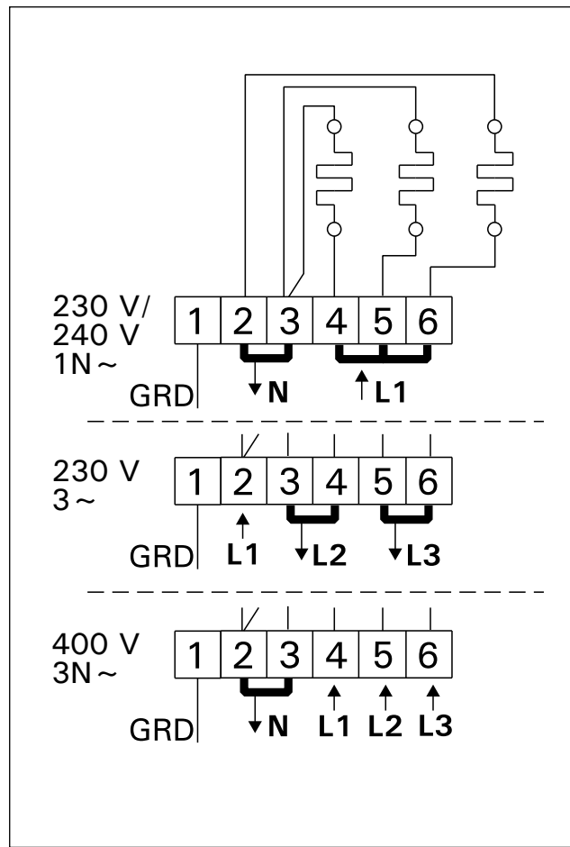
Kuva 11. BC-E-kiukaan sähkökytkennät Bild 11. BC-E-aggregatets elinstallationer
