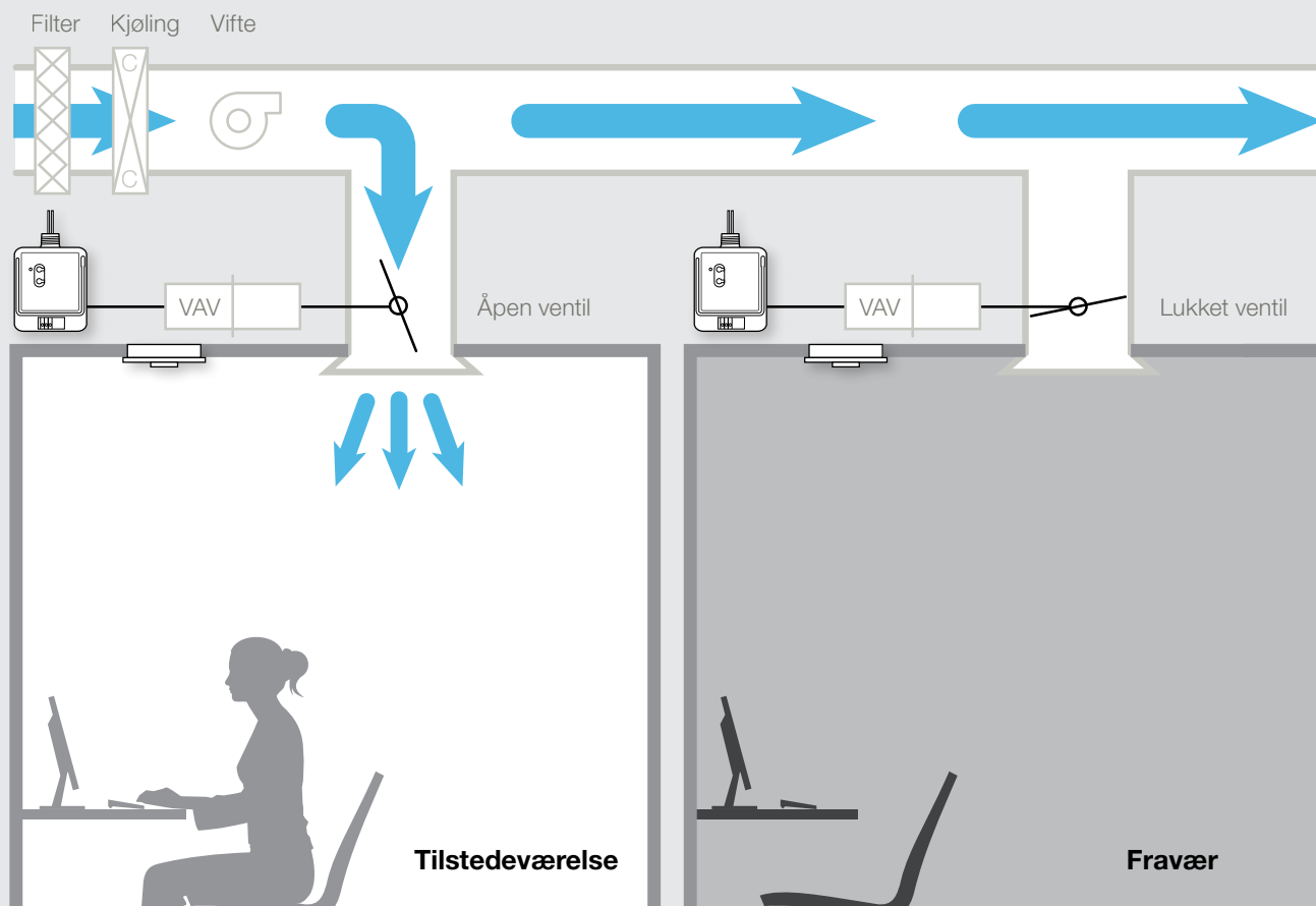
Radio Powr Savr tilstedeværelse/ fraværsensor for takmontering
