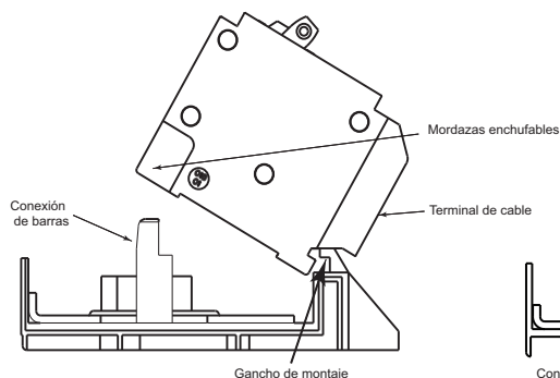
Figura 3: Interruptor automático HOM o HOMT
