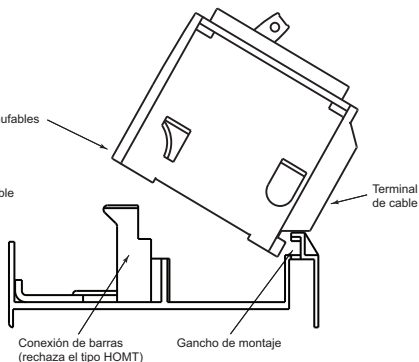
Figura 4: Interruptor automático HOM
