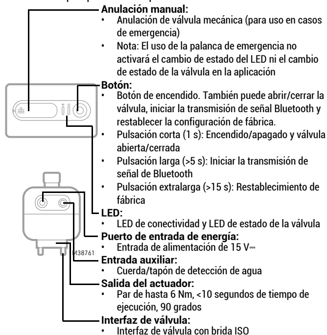
Fig. 2. Componentes
