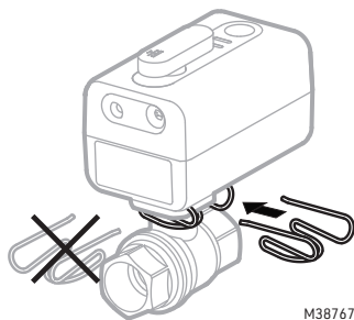
Fig. 4. Connectez la vanne à boisseau sphérique à l'actionneur.
