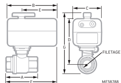
Fig. 7. Schéma dimensionnel.
