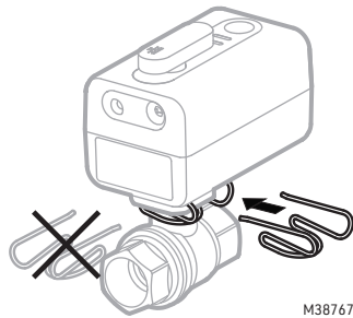
Fig. 4. Conecte la válvula de bola al actuador.
