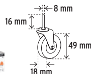
6 Rodajas de polipropileno, con baleros, resistentes a la abrasión, a la deformación y al impacto
