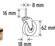
6 Rodajas de nylon, con baleros, resistentes a la abrasión, a la deformación y al impacto
