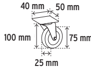
4 Rodajas con balero y 2 con freno manual
