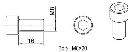
Bolt: M8x20
