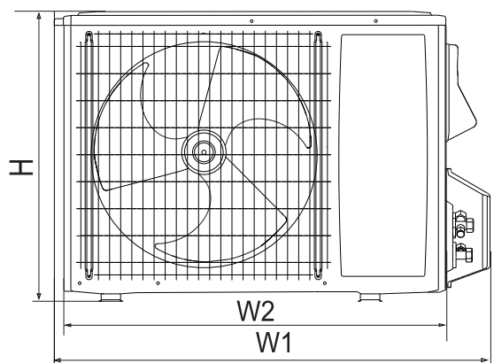
Dimensions de l'unité extérieure
