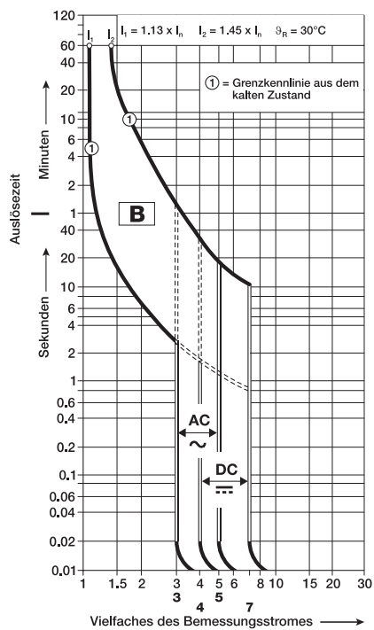
B Charakteristik
