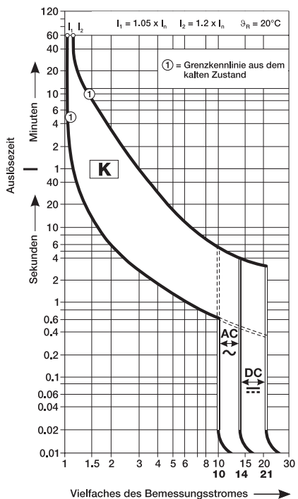
K Charakteristik
