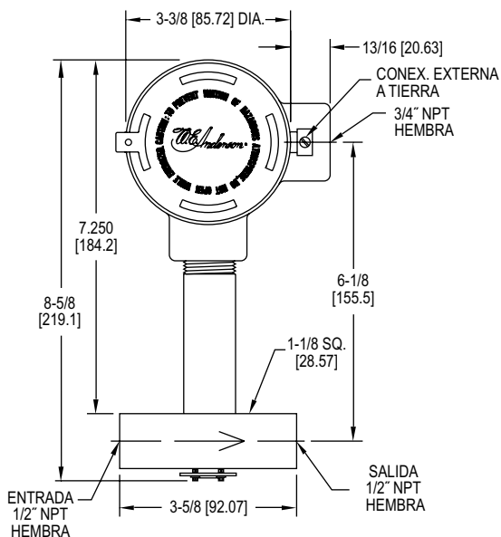
V6 de bajo caudal con caja de conductor CSA, IECEx, ATEX
