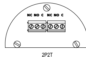
Conexiones terminales CSA, IECEx, cajas ATEX
