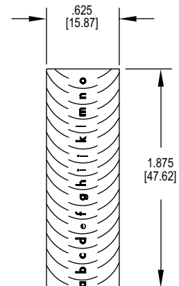
Trimmable vane
