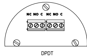
Bornes de raccordement Boîtiers CSA, IECEx, ATEX
