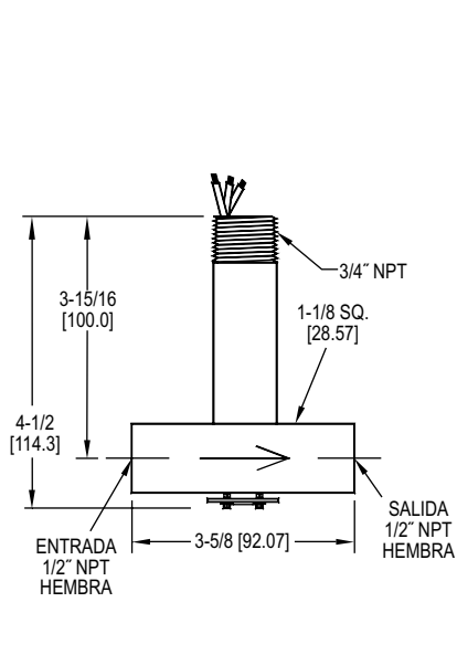
V6 Bajo caudal
