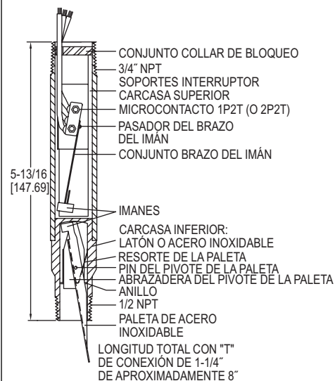
V6 con aleta recortable en campo
