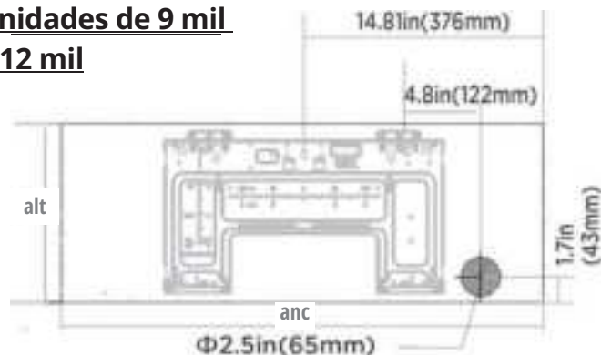
Dimensiones de la unidad interior (anc x alt)
