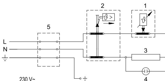
Elektromos bekötés vázlat
