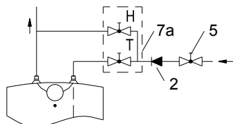
Uzstādīšana zem vannas/izlietnes
