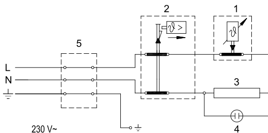
Schéma elektrického připojení
