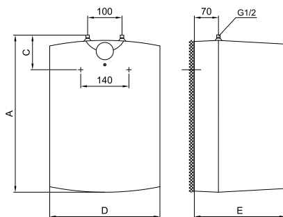
Typ pod umyvadlom
