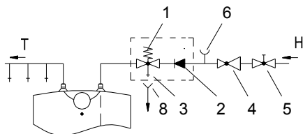
Montavimas po praustuvo / kriaukle
