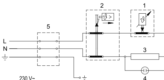
Schemat podłączenia do sieci
