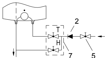
Montavimas virš praustuvo / kriauklės
