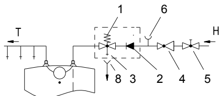
Uzstādīšana zem vannas/izlietnes
