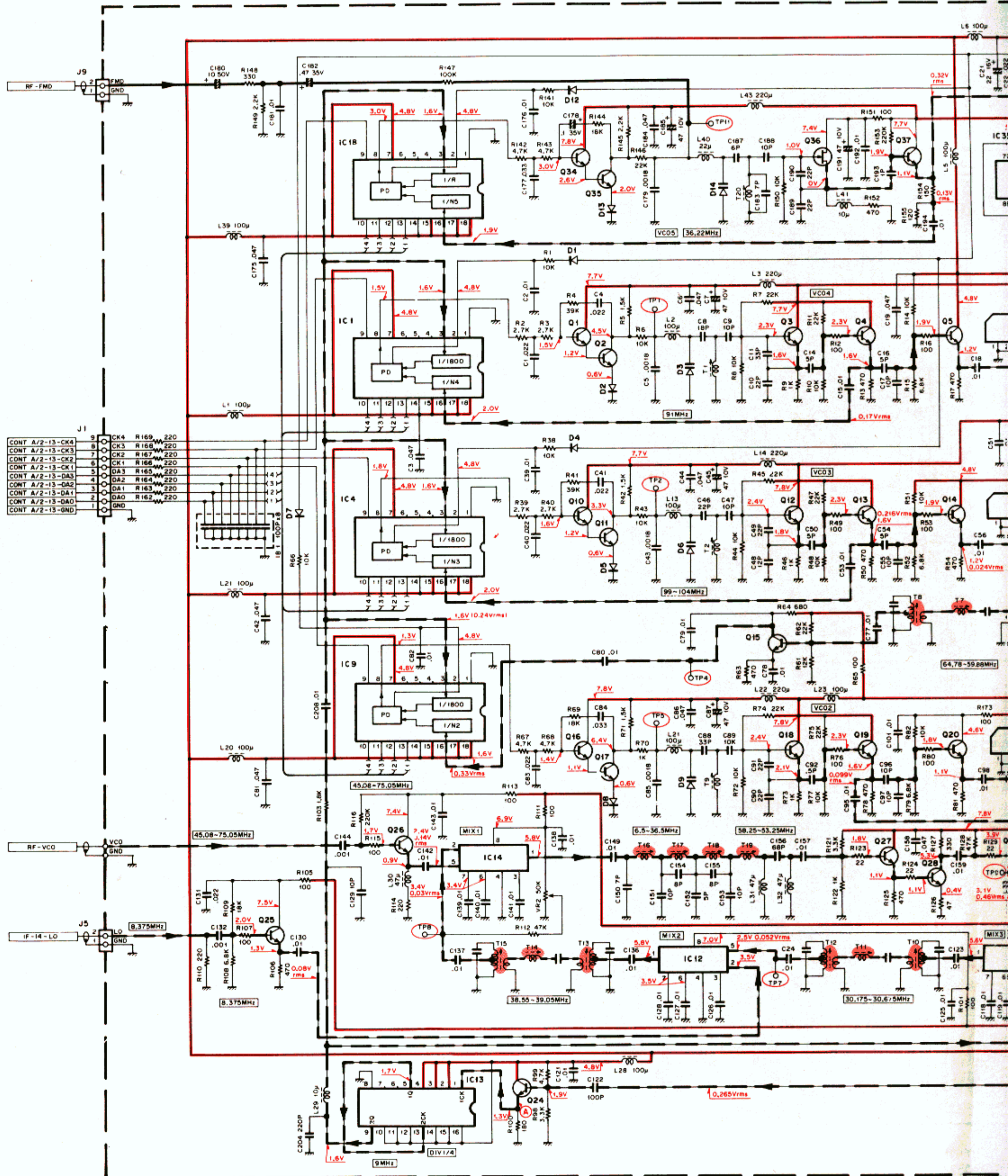
PLL UNIT (X50-2050-00)
