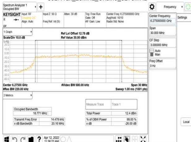
802.11ax_20MHz_Chain0_6275MHz
