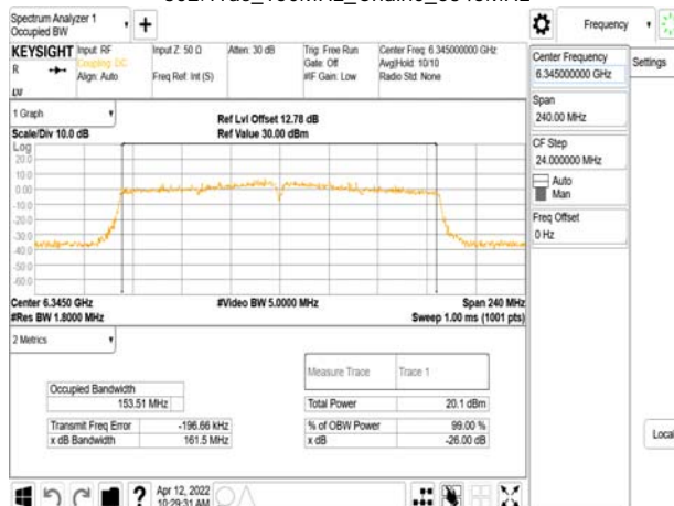
802.11ac_160MHz_Chain0_6345MHz
