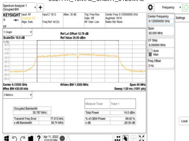
802.11n_40MHz_Chain1_6125MHz
