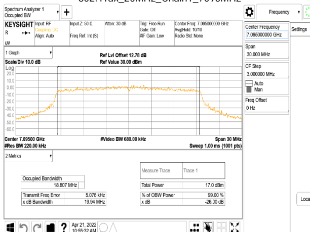
802.11ax_20MHz_Chain1_7095MHz
