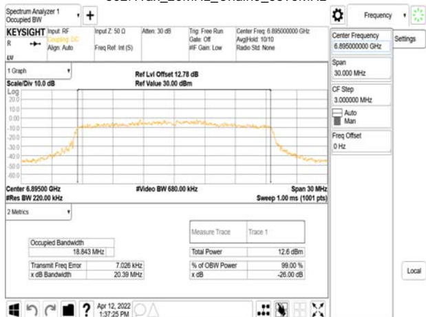
802.11ax_20MHz_Chain0_6895MHz
