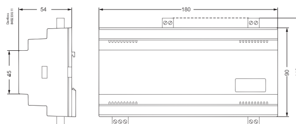
AK-PC 530
