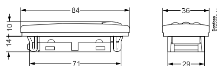
AK-PC 530
