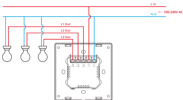
灯具接线示意
