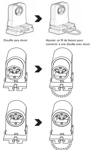
La figure montre comment modifier une douille sans shunt à une douille avec shunt à l'aide d'un fil de liaison.
