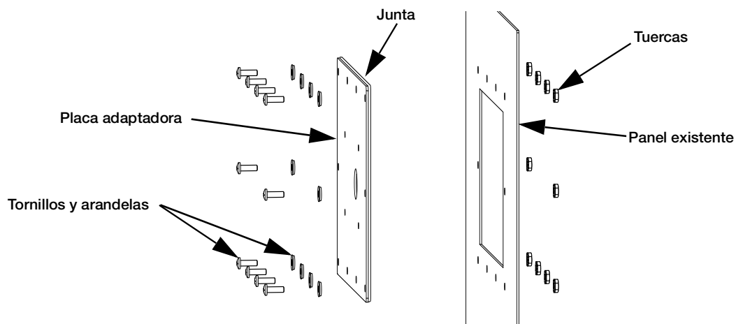
Figura 4. Instalación de la placa adaptadora
