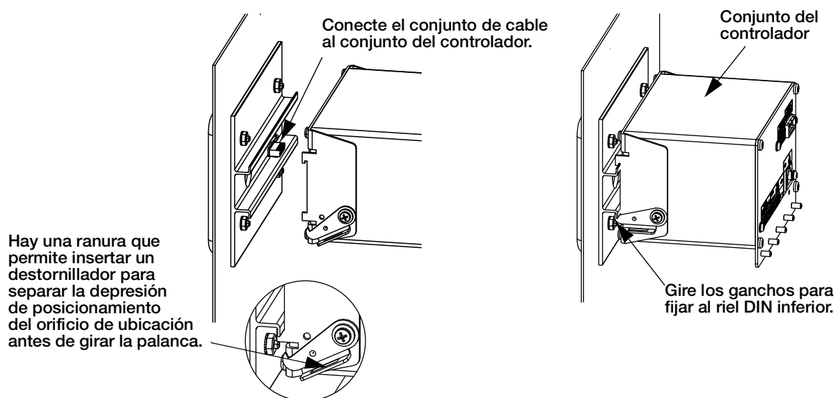
Figura 6. Instalación del conjunto del controlador
