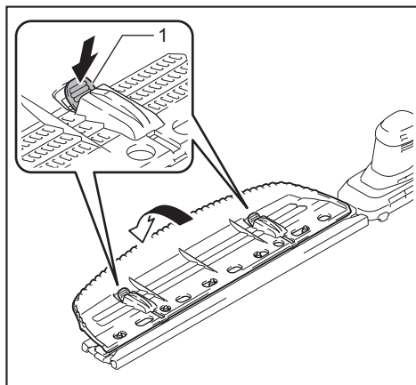
► 1. Lever
