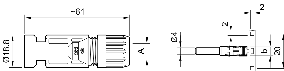
Kupplungsstecker PV-KST4...
