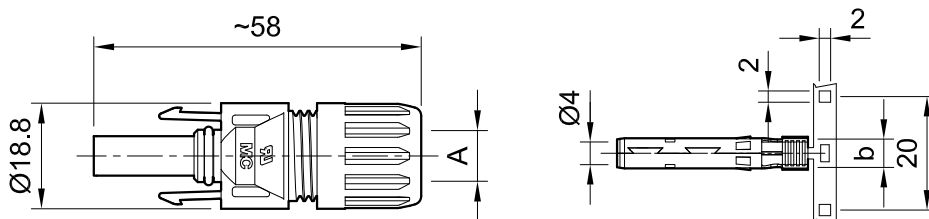
Kupplungsbuchse PV-KBT4...
