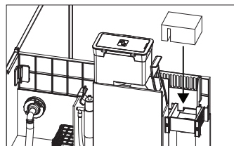
Oberflächenabschäumer/Kamm
