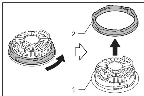
► 1. Fan unit 2. Ring
