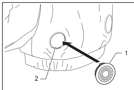
► 1. Fan unit 2. Hole
