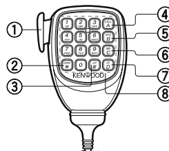
Micrófono DTMF
