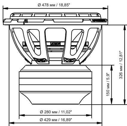
DB-4518R D1/D2
