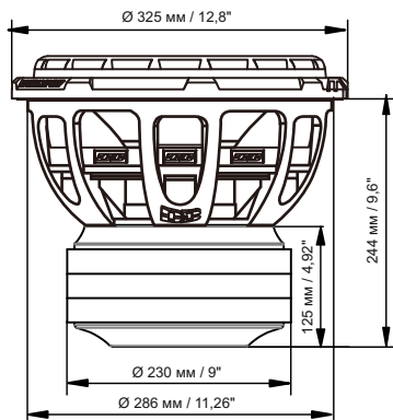
DB-4515R D1/D2
