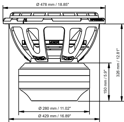
DB-4518R D1/D2
