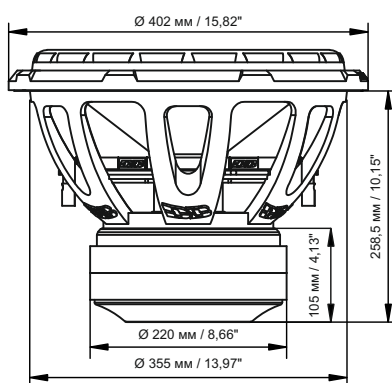
DB-3015R D1/D2
