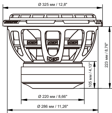
DB-3012R D1/D2
