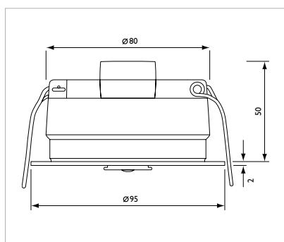
Boîtier de montage en surface OccuSwitch LRM1070 Dimensions en mm.
