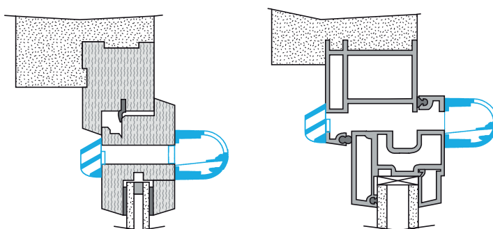
Coupe entrée d'air EA
