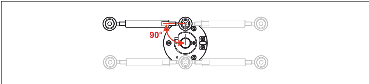
Abbildung 13: Gelenkkopfstab – Montagevarianten
