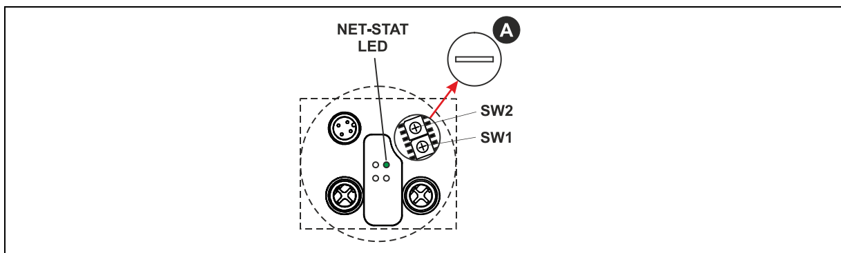
Abbildung 5: Zugang Drehschalter
