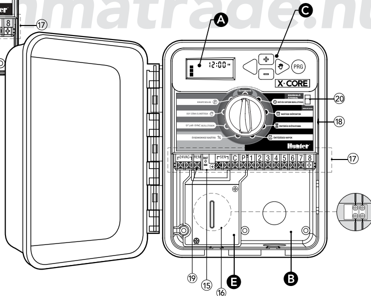
Kültéri típus (beépített transzformátorral)
