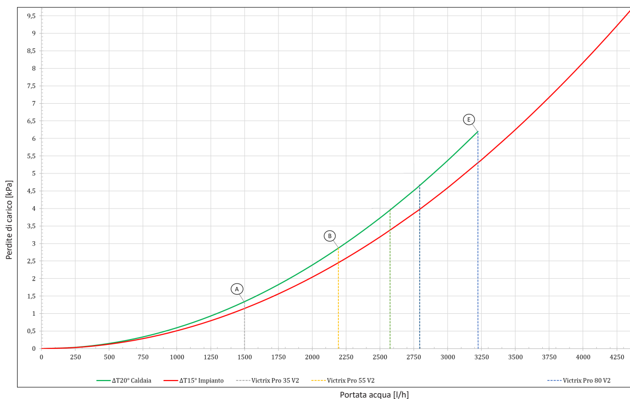
Grafico perdite di carico kit scambiatore a piastre caldaia singola VICTRIX PRO 35-55-80 V2 \Delta T_{20^\circ} Primario / \Delta T_{15^\circ} Secondario
