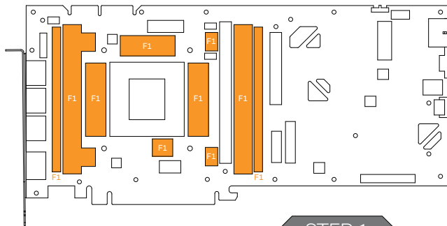
F1 Thermal Pad - 120 x 16 x 1.0 mm
