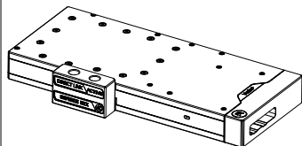
EK-Quantum Vector² FTW3 RTX 3090 Ti ABP Set D-RGB
