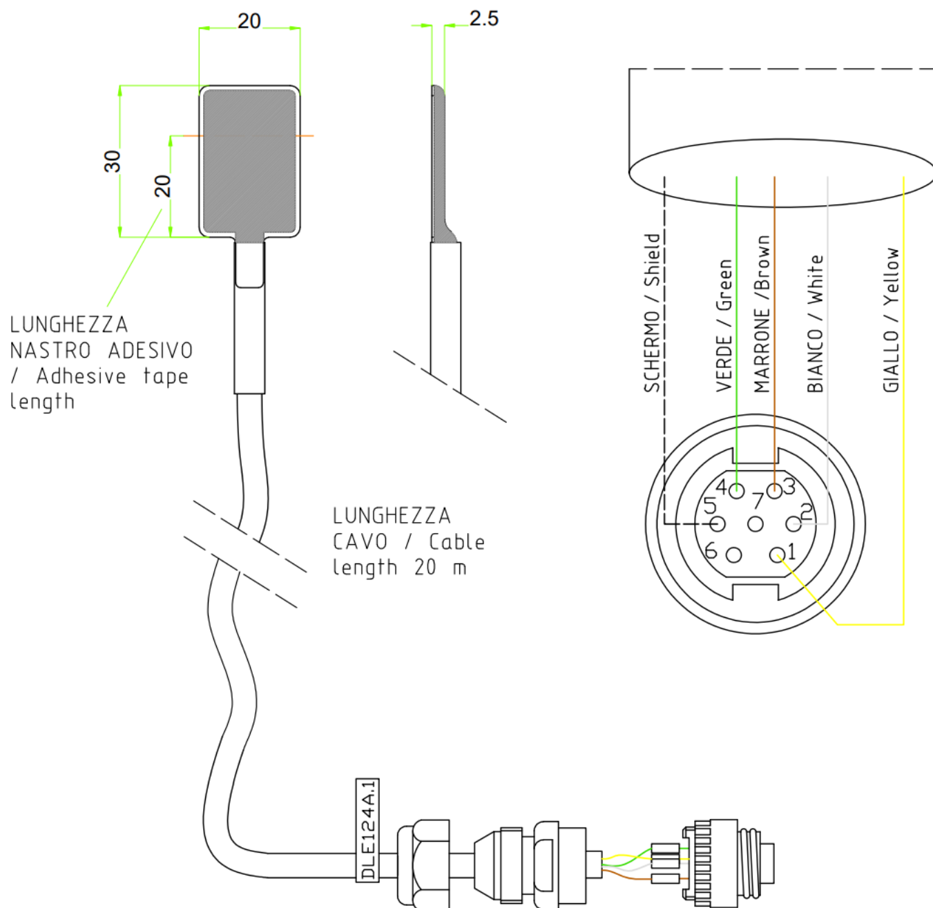
SCHEMA DI COLLEGAMENTO Pt100 / Connection diagram of P1100
